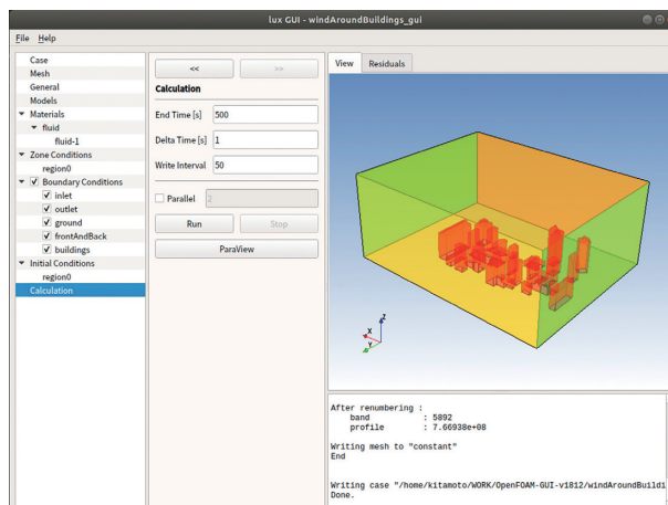
図3：GUI“luxgui”による計算設定
