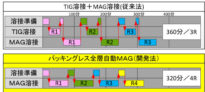
図6 シールド内配管工事 タイムサイクル (実績比較：500A×12.7mmt X60)
