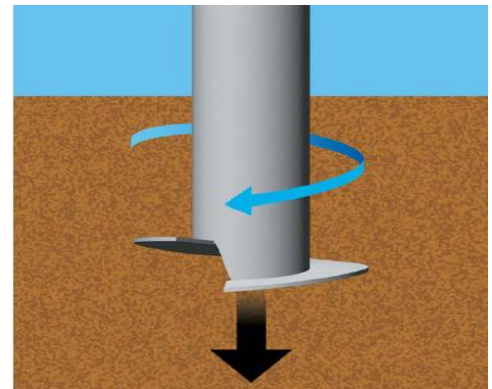
図1 回転による貫入施工
