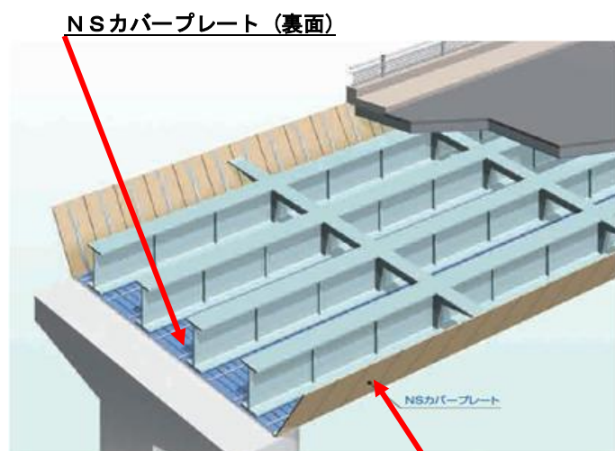
【NSカバープレートの構造】 NSカバープレート(裏面) NSカバープレート(側面)
