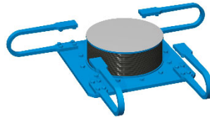
ダンパー4本タイプ(T型)
