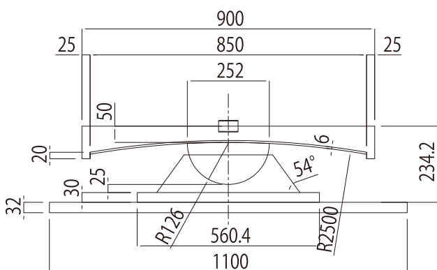
断面図
